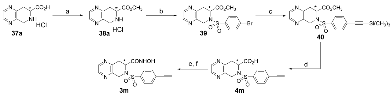
Scheme 8. (Method D). Reagents: (a) \text{SOCl}_2 , \text{MeOH} ; (b) bromobenzenesulfonyl chloride, \text{Et}_3\text{N} ; (c) \text{Et}_3\text{N} , \text{Ph}_3\text{P} , \text{CuI} , trimethylsilylacetylene; (d) \text{KOH} aq; (e) \text{ClCOCOCl} ; (f) \text{H}_2\text{NOH} aq.
